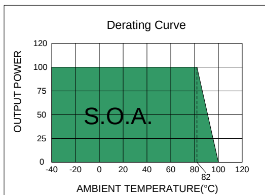
CNC10HW-2415S、CNC10HW-2415D
