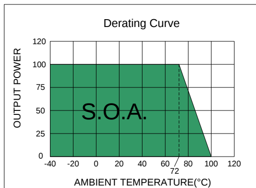
CNC10HW-1205S、CNC10HW-1205D
