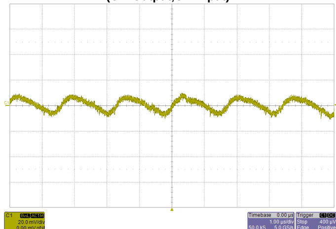
Noise V_{IN}=5V , I_O=6A , 5~20MHz Bandwidth
