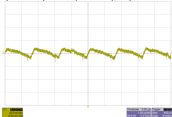
Noise V_{IN}=12V , I_O=6A , 5~20MHz Bandwidth
